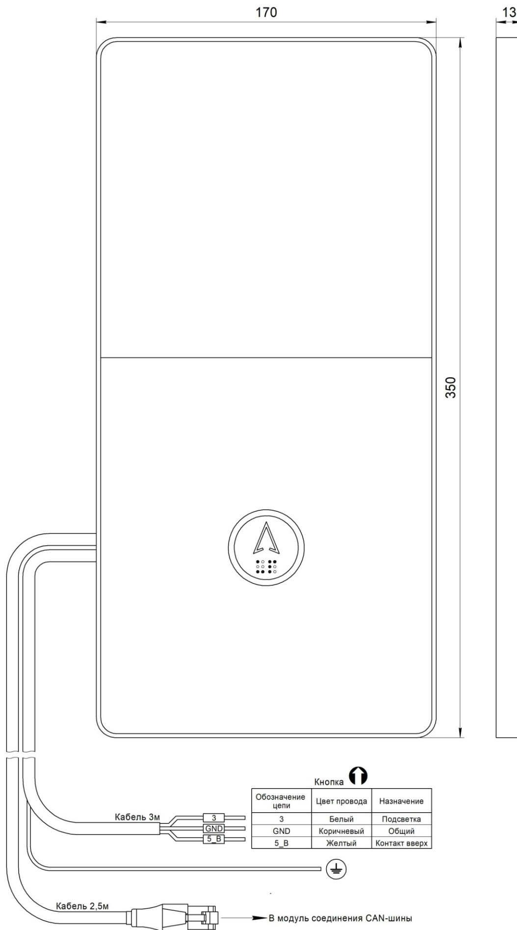
Рис.1 Внешний вид, габаритные и установочные размеры Вызывного поста МАЛАХИТ (жгут RJ45) НШЕК.468381.017
